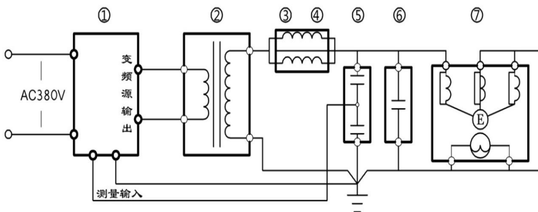
发电机耐压试验接线图
